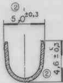
CORTE - AA
